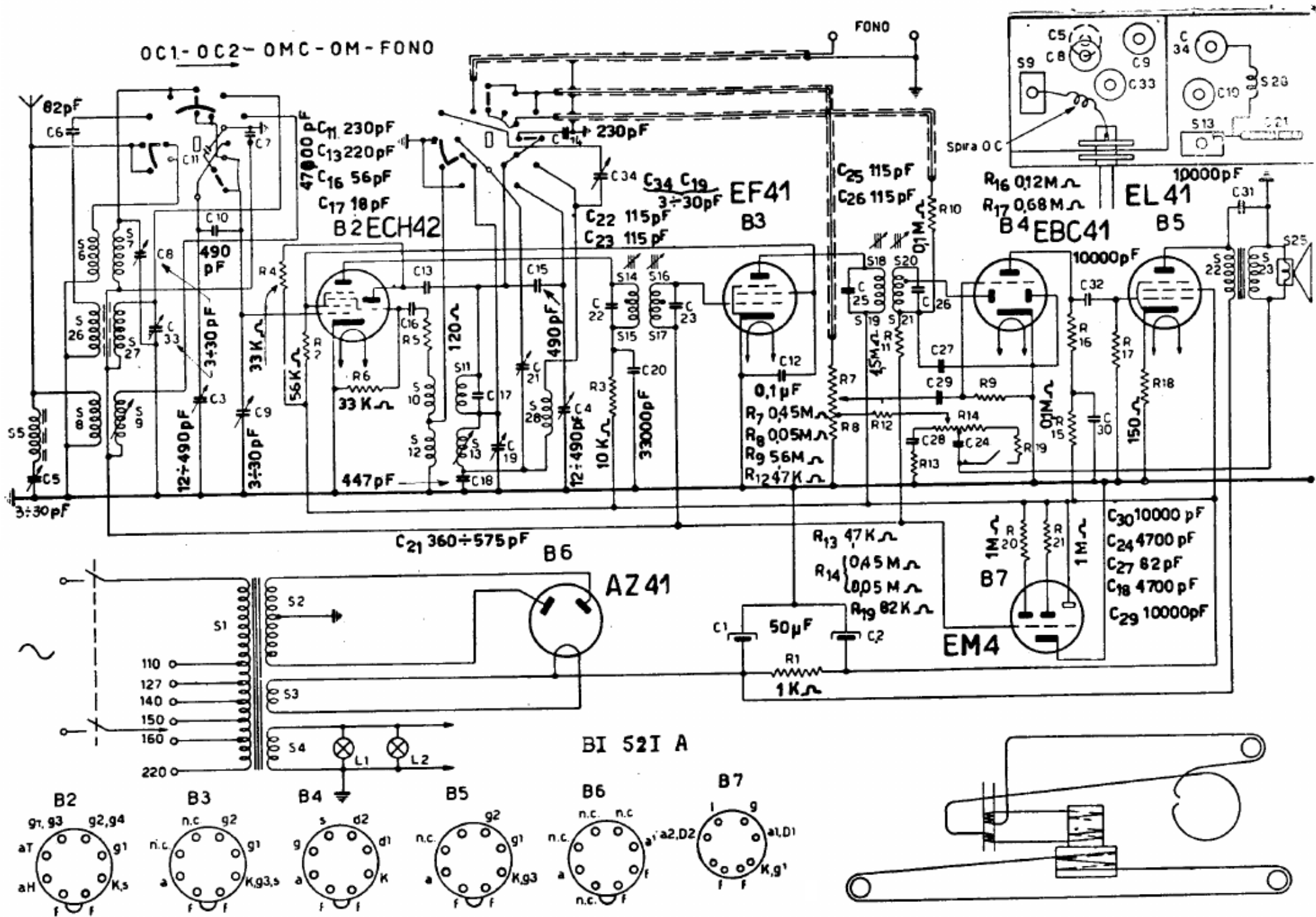
PHILIPS RADIO - Mod. BI 521 A. Quattro gamme d'onda: onde medie da 1630 a 517 kc/s; onde medie corte da 3,1 a 1,6 Mc/s e due gamme onde corte, compresa quella per pescherecci. Media frequenza 468 kc/s. Corrente anod. totale 60 mA. Consumo 44 watt.
